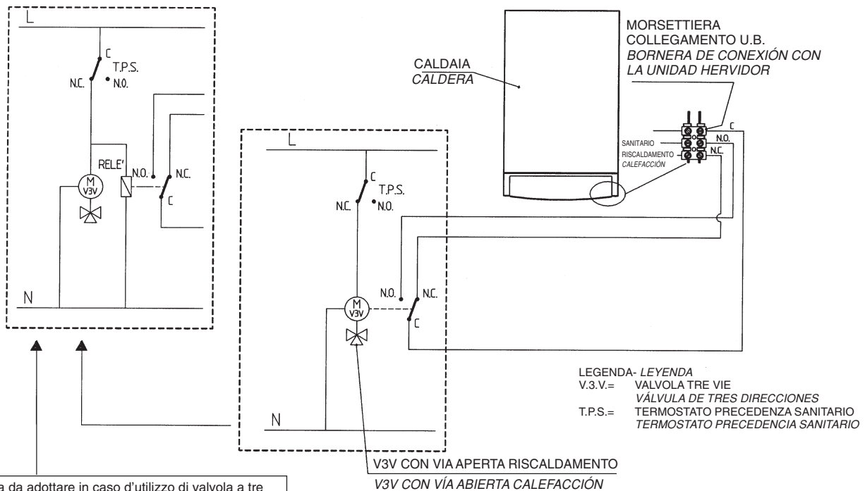
SCHEMA CON VALVOLA A TRE VIE CON RITORNO A MOLLA DIAGRAMA CON VÁLVULA DE TRES VÍAS CON RETORNO POR MUELLE
