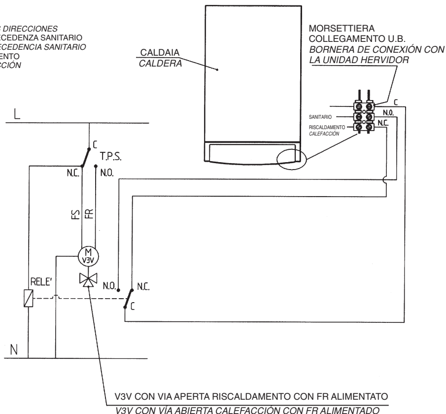
SCHEMA CON VALVOLA A TRE VIE A DOPPIA ALIMENTAZIONE DIAGRAMA CON VÁLVULA DE TRES VÍAS DE DOBLE ALIMENTACIÓN
